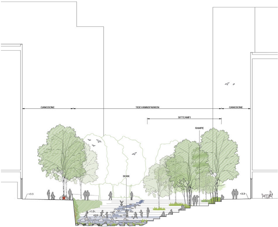
Snitt AA. Tidevannsparken
