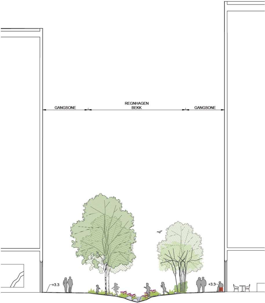
Snitt AA. Regnhagen
