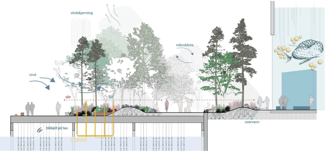
Snitt AA. Havnepromenaden
